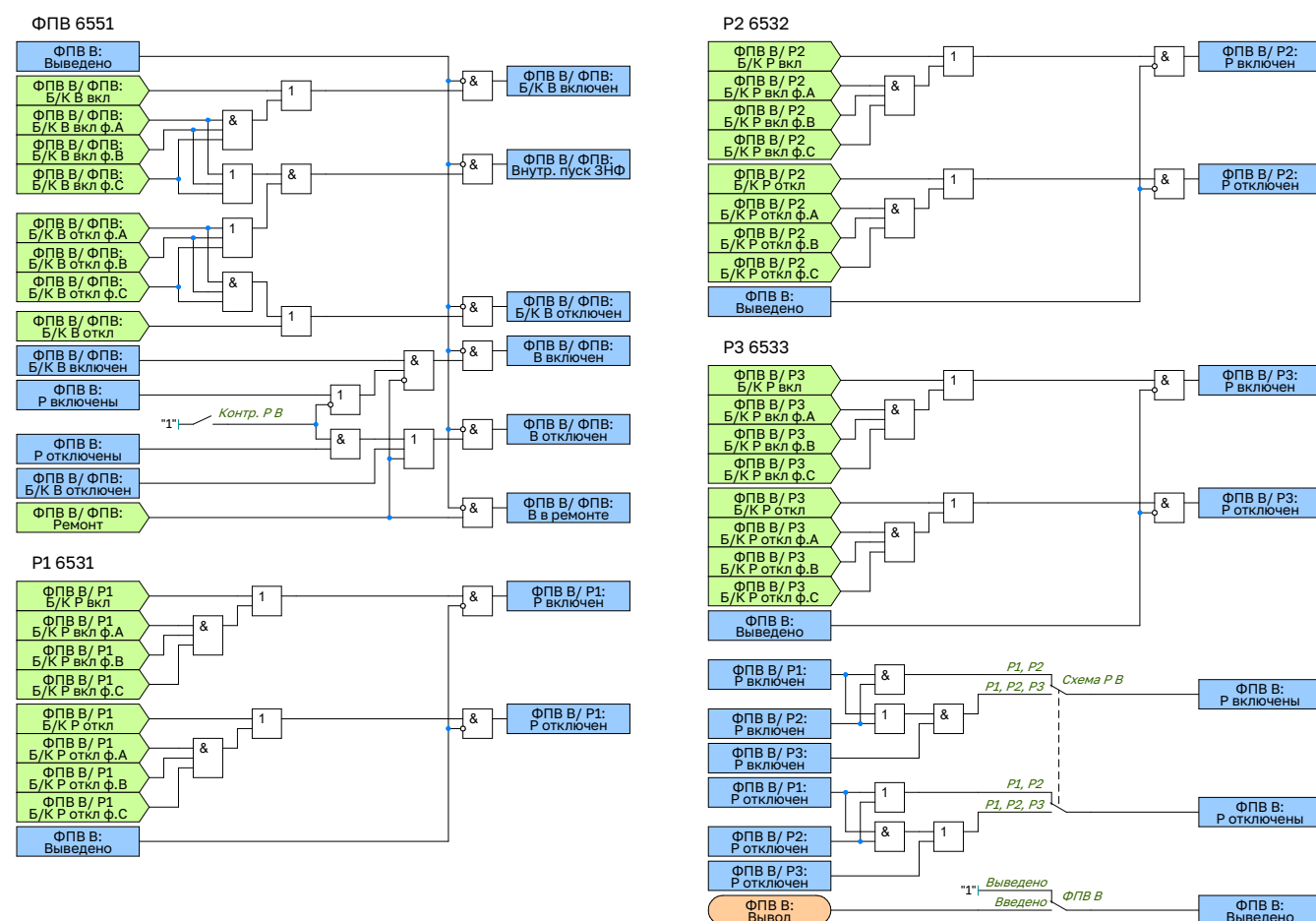
Рисунок 2.72 – Функциональная схема логики ФПВ В1
