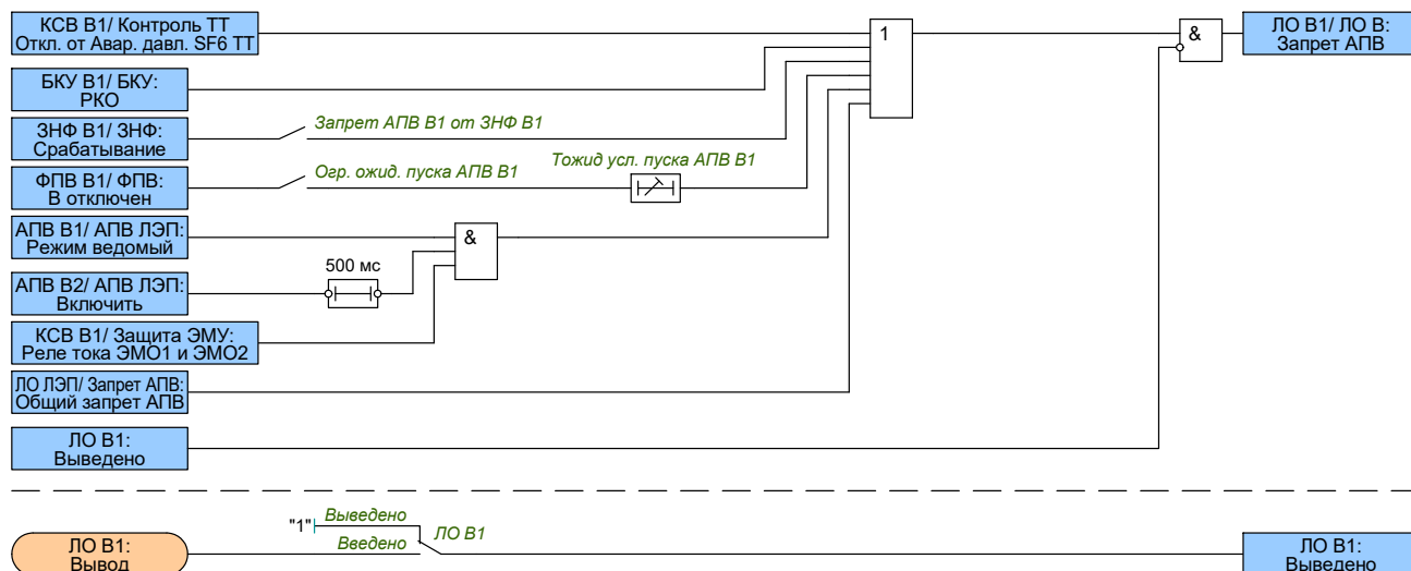
Рисунок 2.70 – Функциональная схема запрета АПВ В1
