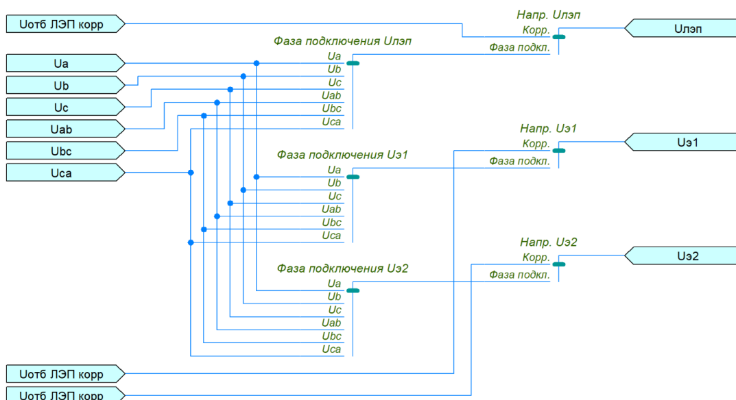
Рисунок 2.71 – Функциональная схема настройки аналоговых значений U_{лэп} , U_{э1} , U_{э2}
